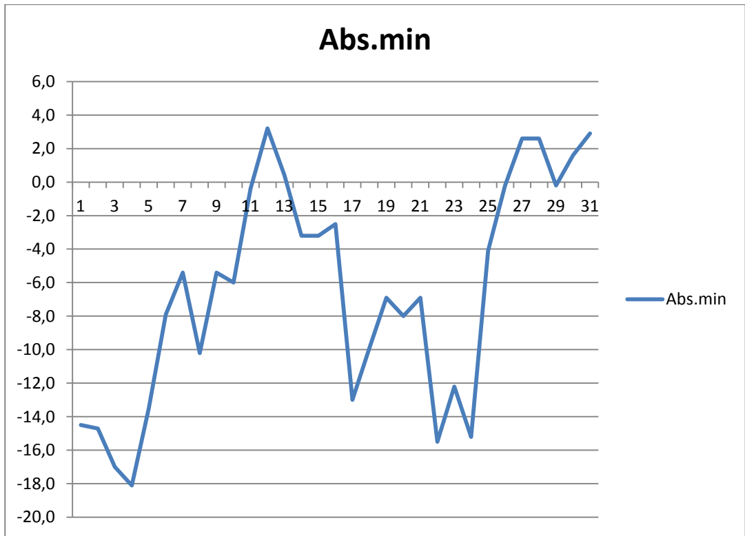
Графік абсолютної мінімальної добової температури повітря °C
