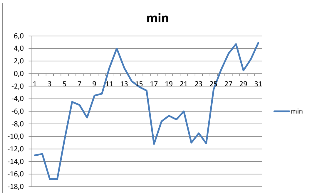
Графік мінімальної добової температури повітря °С
