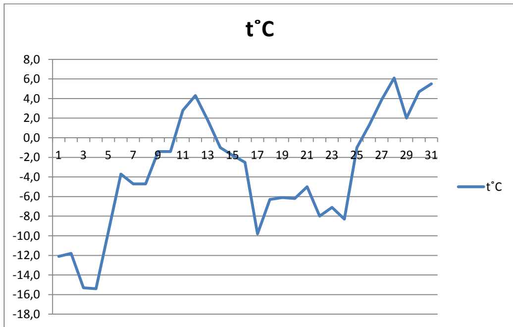
Графік середньої добової температури повітря °С
