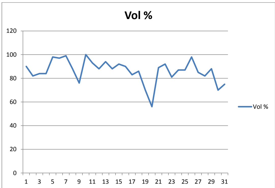
Графік добового ходу відносної вологості повітря в %
