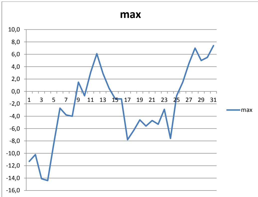
Графік максимальної добової температури повітря °C
