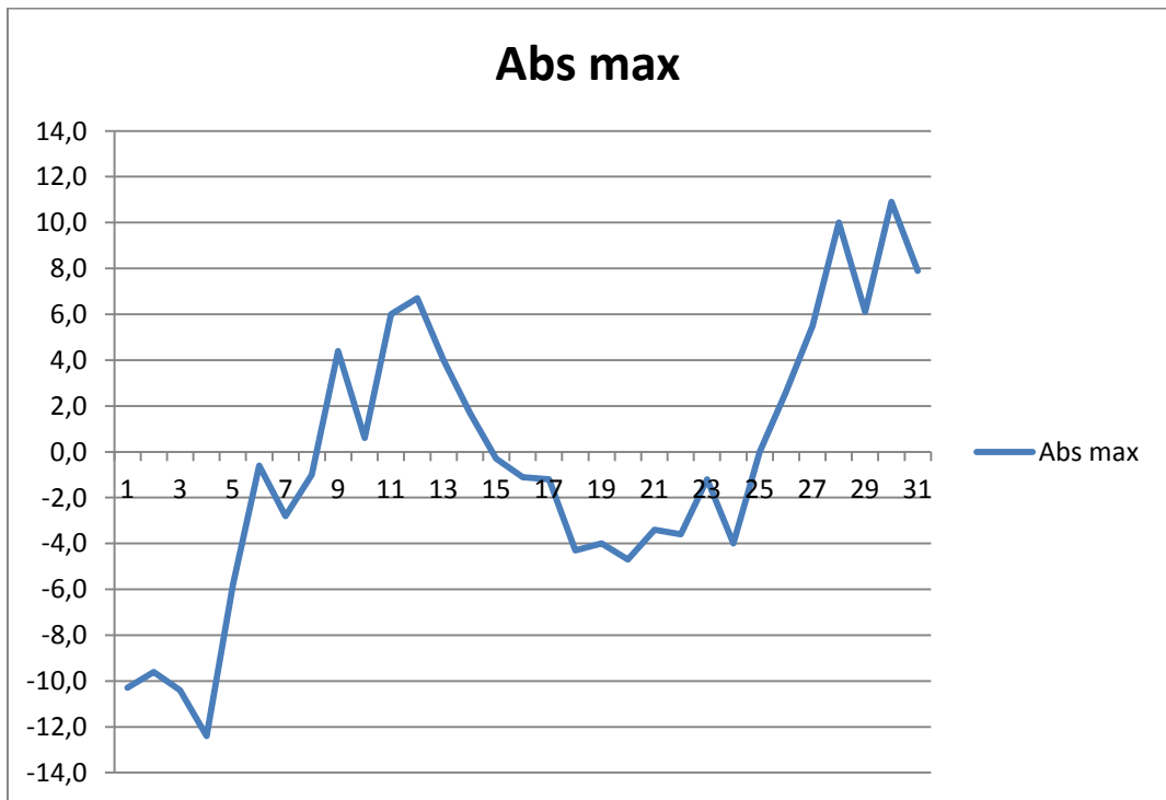
Графік абсолютної максимальної добової температури повітря °C
