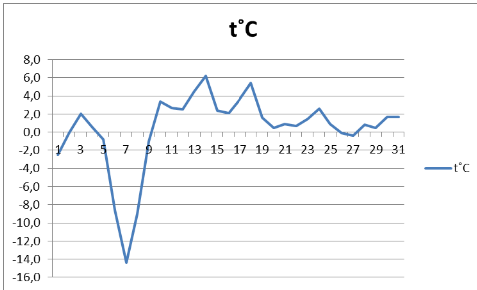
Графік середньої добової температури повітря °C
