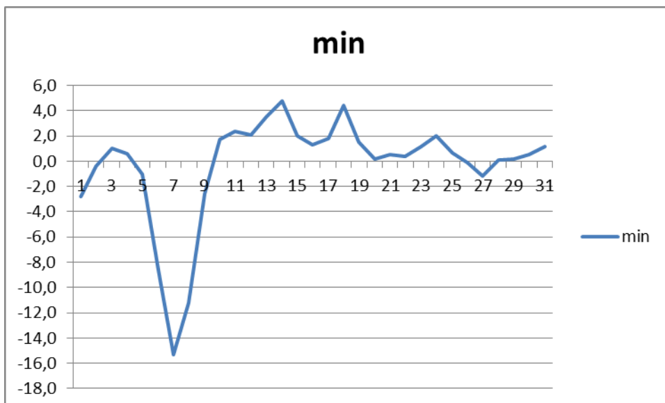
Графік мінімальної добової температури повітря °C
