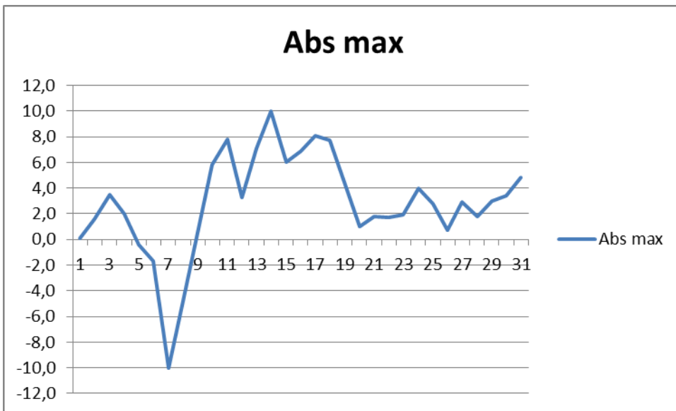
Графік абсолютної максимальної добової температури повітря °С
