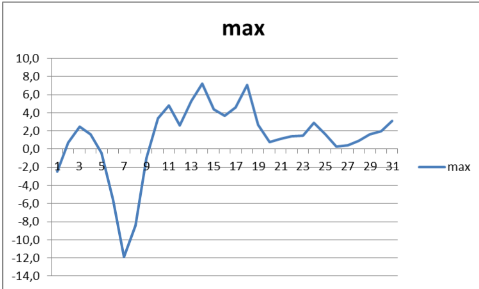
Графік максимальної добової температури повітря °С
