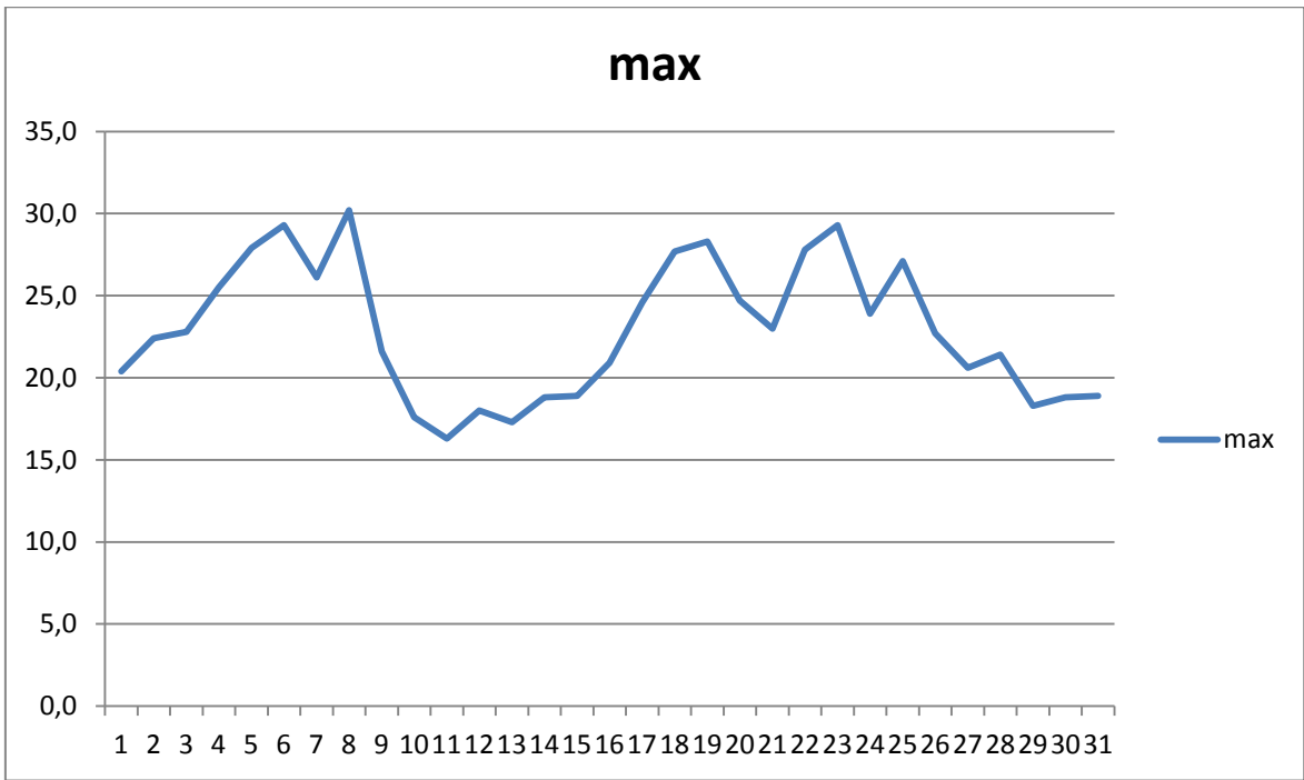
Графік максимальної добової температури повітря °C
