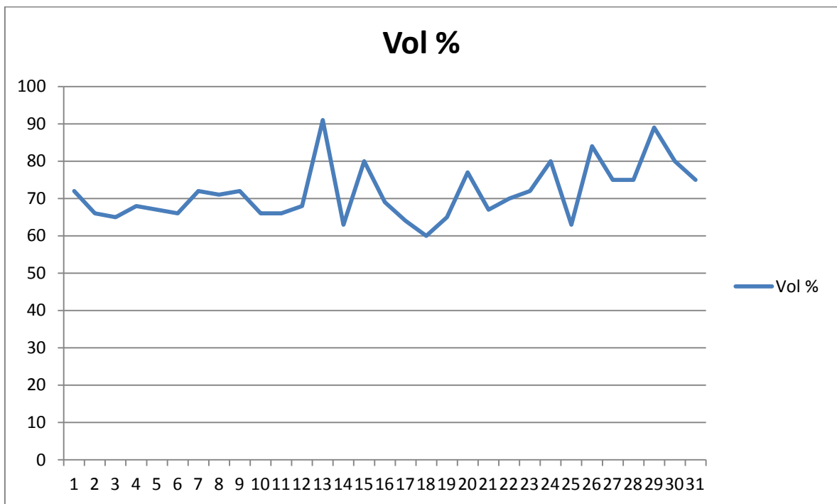
Графік добового ходу відносної вологості повітря в %
