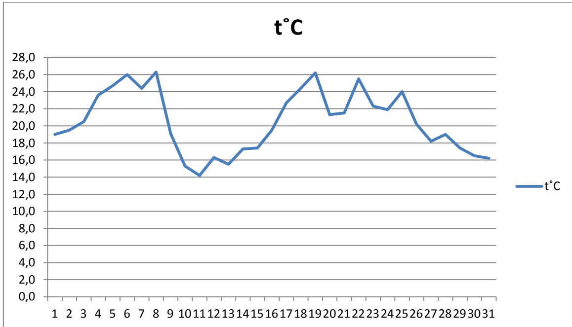
Графік середньої добової температури повітря °C
