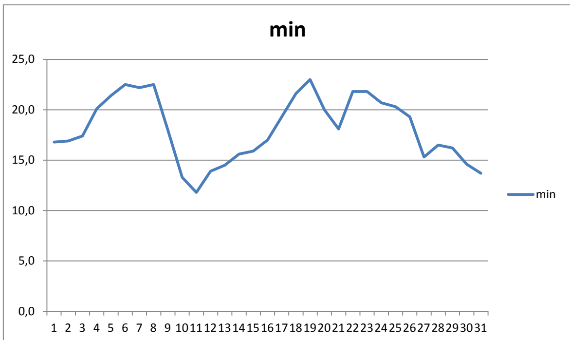
Графік мінімальної добової температури повітря °C
