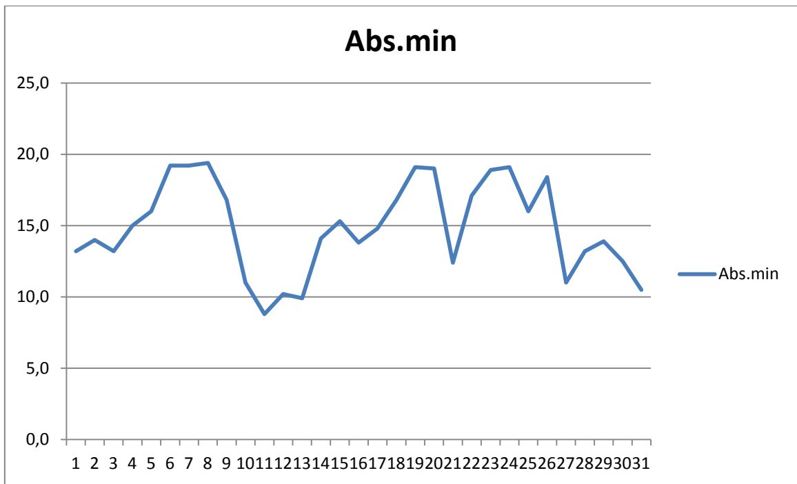
Графік абсолютної мінімальної добової температури повітря °С
