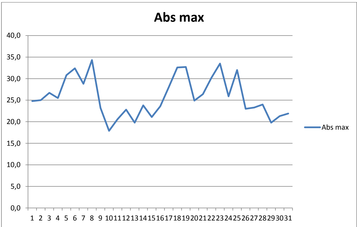
Графік абсолютної максимальної добової температури повітря °C
