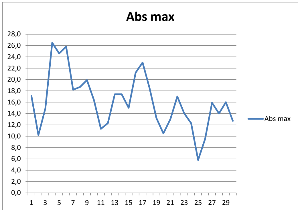
Графік абсолютної максимальної добової температури повітря °С
