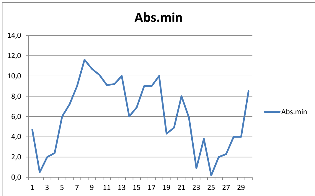
Графік абсолютної мінімальної добової температури повітря °C
