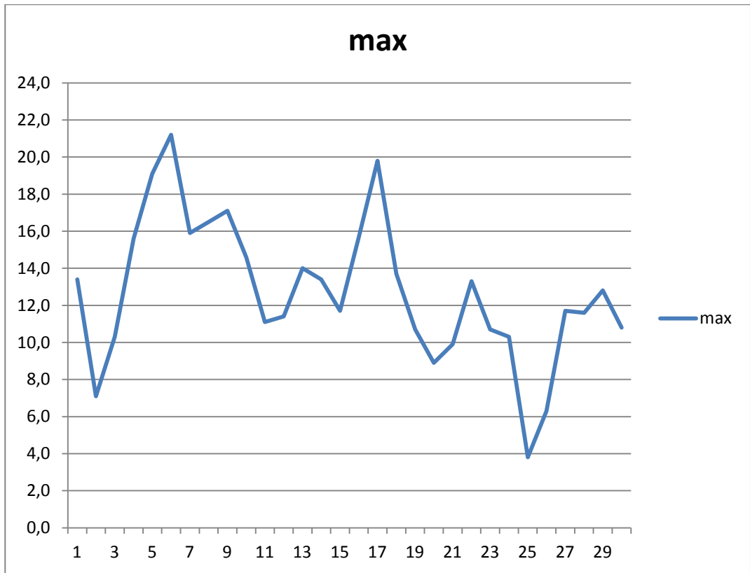
Графік максимальної добової температури повітря °С
