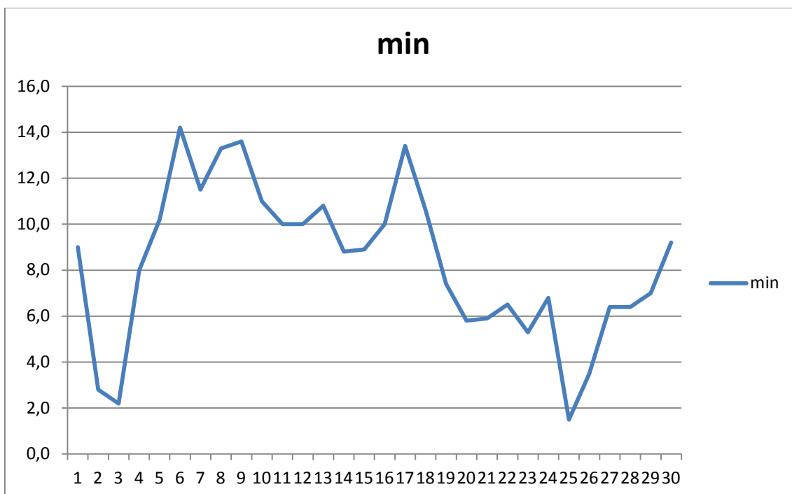
Графік мінімальної добової температури повітря °С
