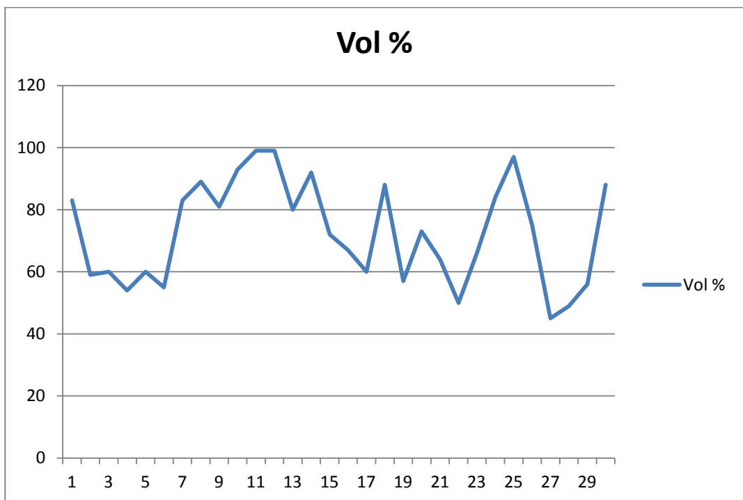
Графік добового ходу відносної вологості повітря в %
